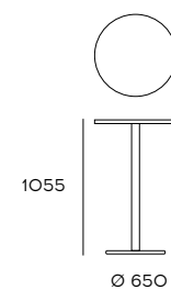
Tavolo alto tondo high round table, runder Hochtisch
