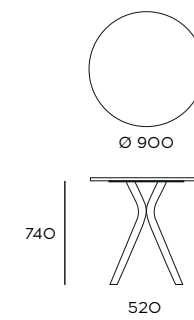
Tavolo tondo a gambe centrali round table, rund Tisch
