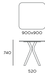
Tavolo quadrato a gambe centrali square table, quadratischer Tisch
