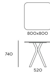
Tavolo quadrato a gambe centrali square table, quadratischer Tisch
