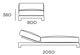
Letfino singolo Java sunlouger, sonnenliege (1 Person)
