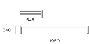
Letfino senza braccioli sunlounger without armrests, Sonnenliege ohne Armlehnen
