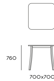
Tavolo table, tisch
