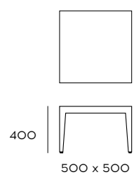
Tavolino basso Bizet coffee table, kaffeetisch
