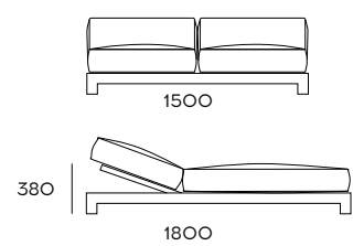
Letfino doppio Java sunlouger, Sonnenliege (2 Personen)
