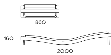
Letfino sun lounger, sonnenliege
