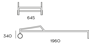
Letfino con braccioli sunlounger with armrests, Sonnenliege mit Armlehnen
