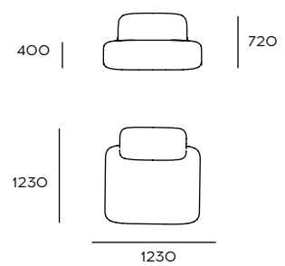
Poltrona senza braccioli slipper chair, Sessel ohne Armlehnen
